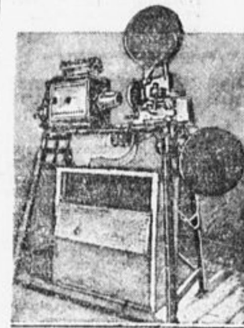
Проекционный аппарат «Тагетон»
